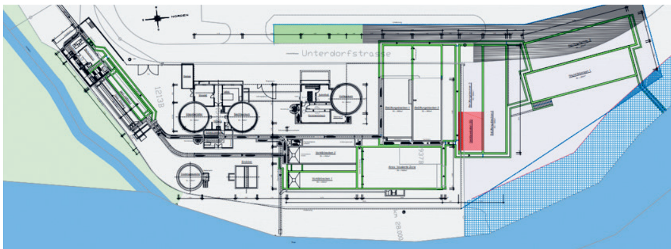
Variante Vorprojekt Zusammenschluss ARA Ganterschwil und ARA Bütschwil
