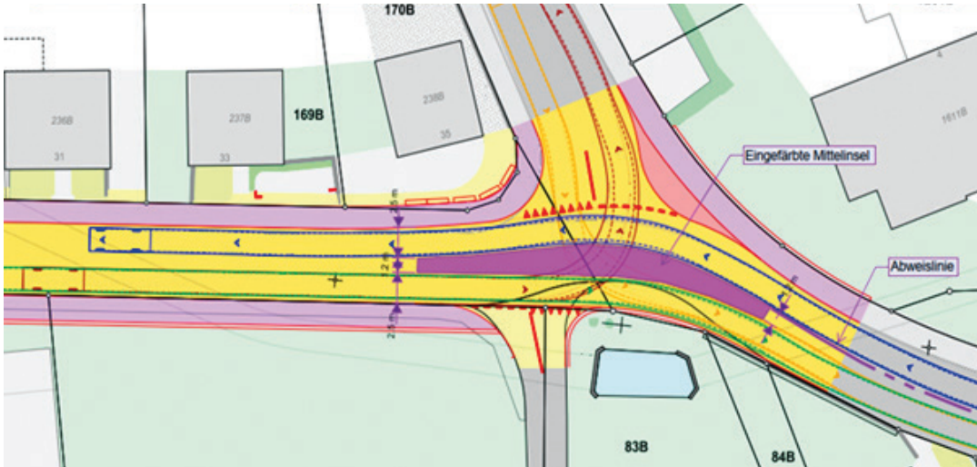
Projektanpassungen Ottilienstrasse (Knoten Mosnangerstrasse)
